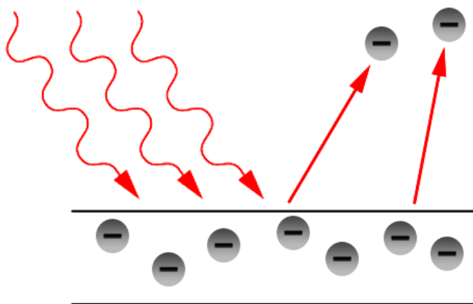
Vonkajší fotoelektrický jav
