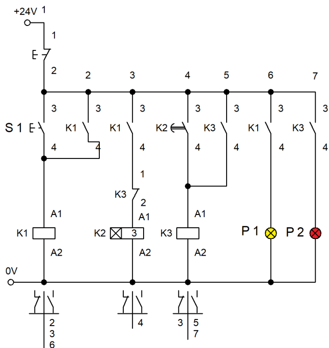
Schéma zapojenia a stavový diagram vytvorené v programe FluidSim
