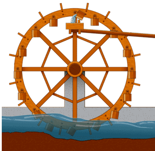
Princíp norie
