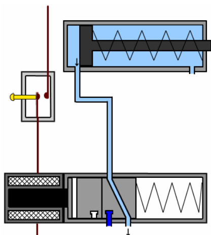
Riadenie 3/2-cestným posúvačovým e-ventilom
