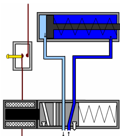
Riadenie 5/2-cestným posúvačovým e-ventilom
