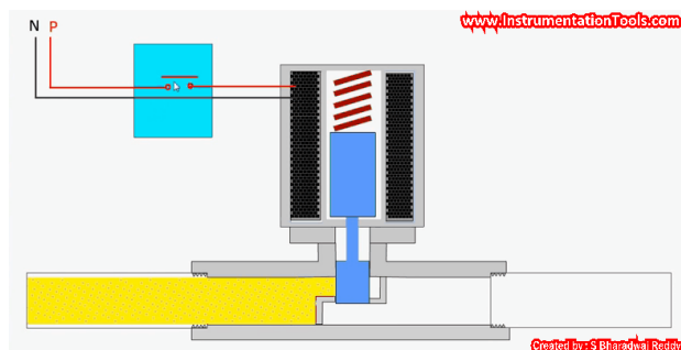
Riadenie sedlovým e-ventilom
