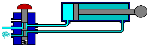
Dvojčinný valec
