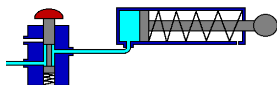
Jednočinný valec
