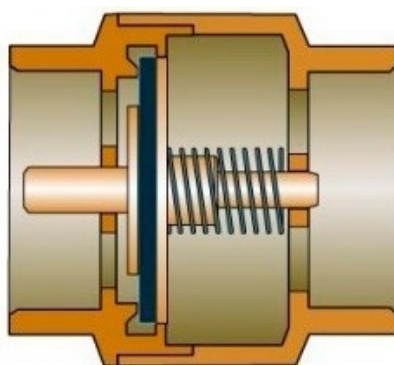
Jednosmerný ventil: nepriepustný smer, priepustný smer.
