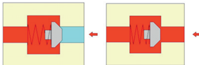
Jednosmerný ventil: nepriepustný smer, priepustný smer.
