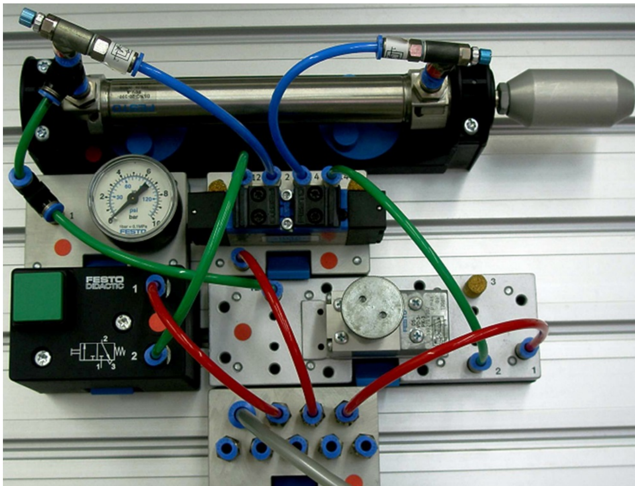
Ukážka zapojenia v školskej praxi Kombinácie ventilov (spájané ventily)
