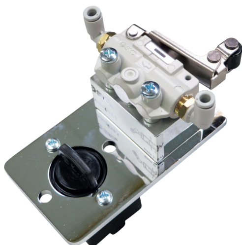
3/2-cestné pneumatické ventily
