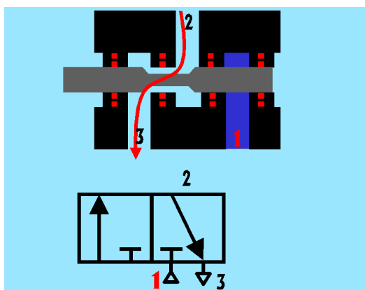
Princíp činnosti
