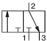
3/2-cestný ventil v základnej polohe uzatvorený NC
