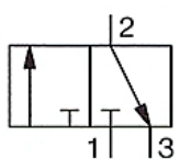
3/2-cestný ventil v základnej polohe uzatvorený
