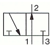
3/2-cestný ventil v základnej polohe otvorený
