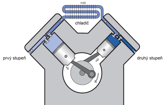
Dvojestupňový piestový kompresor s chladičom vzduchu
