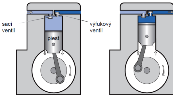
Jednostupňový piestový kompresor
