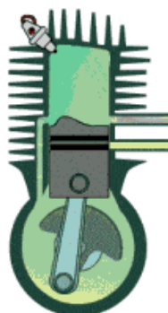
Dvojdobý motor
