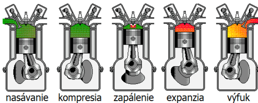
Pracovný cyklus štvordobého motora
