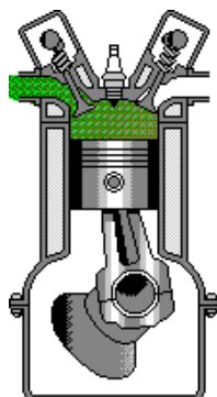
Štvordobý motor
