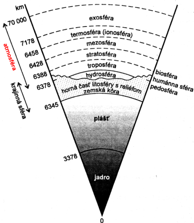
Vertikálny prierez Zemou
