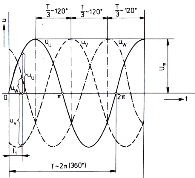
Časový diagram napätí
