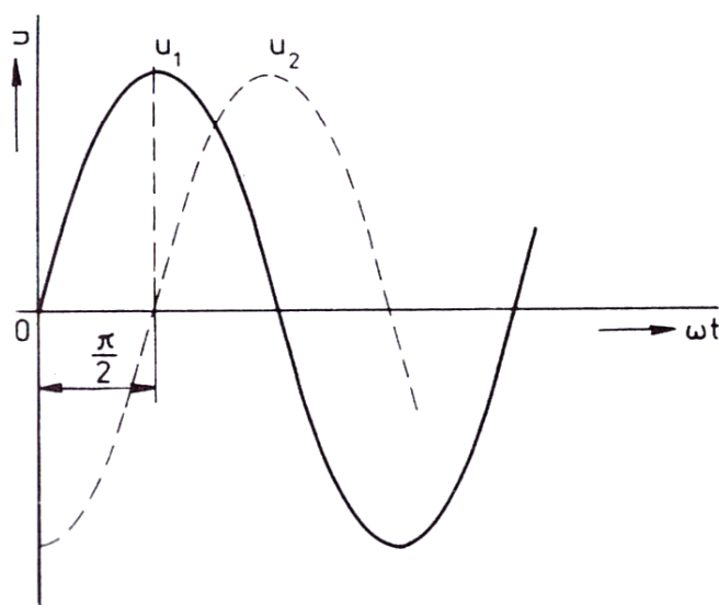
Priebeh 2-fázového napätia
